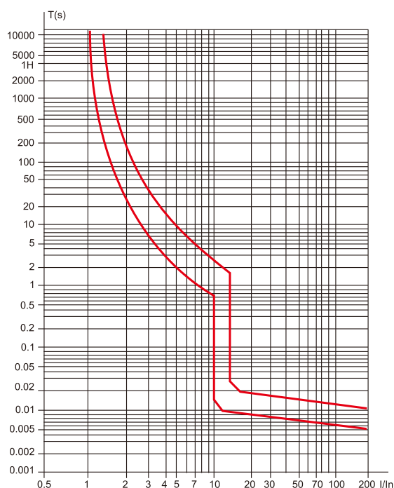
FTB21 (D) 型脱扣曲线
