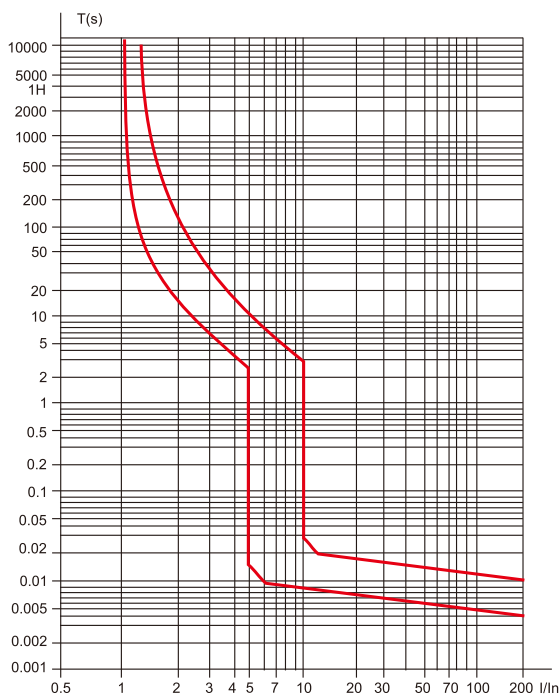
FTB21 (C) 型脱扣曲线
